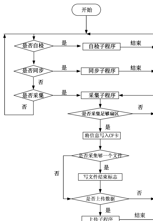
图 6 数字采集模块软件流程图
