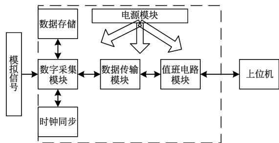
图 2 数字采集与存储单元硬件组成
