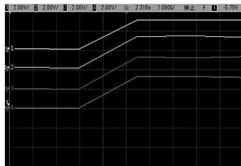
图 11 同步后采集触发秒脉冲
