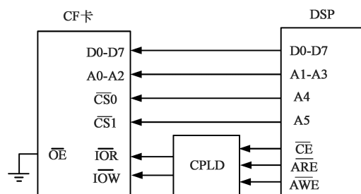
图 5 CF 卡与 DSP 连接示意图
