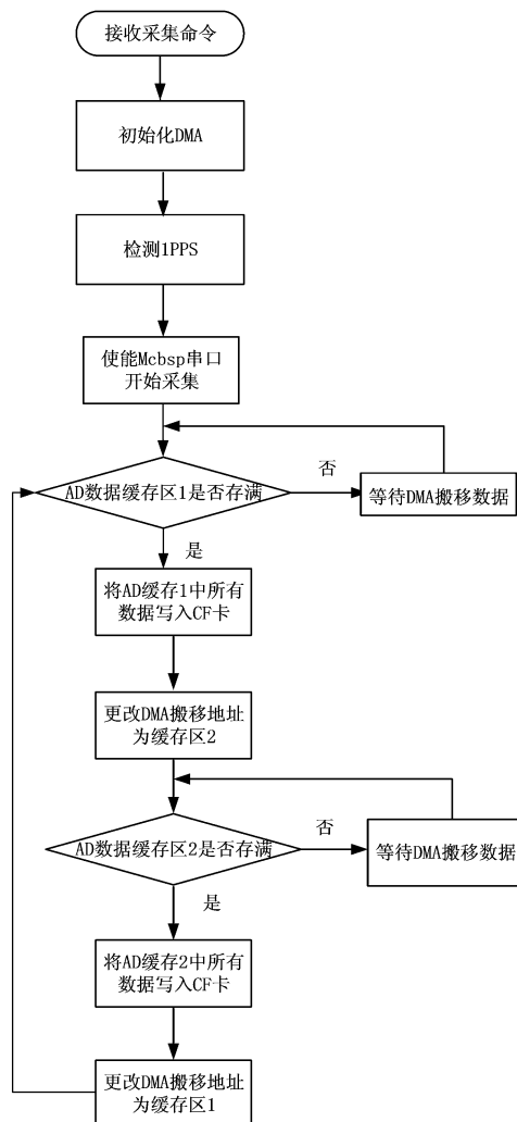
图9 数据采集与存储流程图
