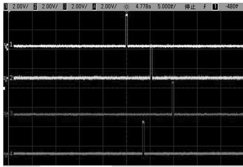
图 10 同步前触发秒脉冲
