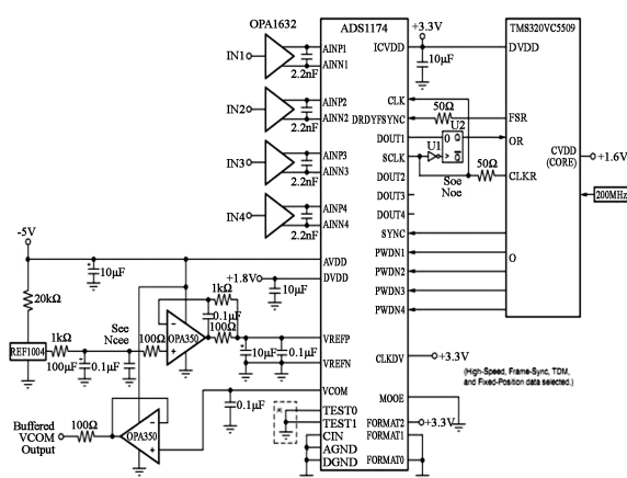
图 3 数字采集模块原理图
